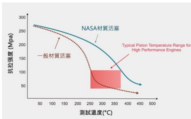
NASA 材質與一般材質高溫下強度比較
